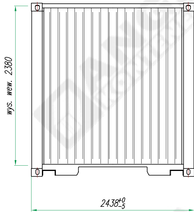
Widok C
