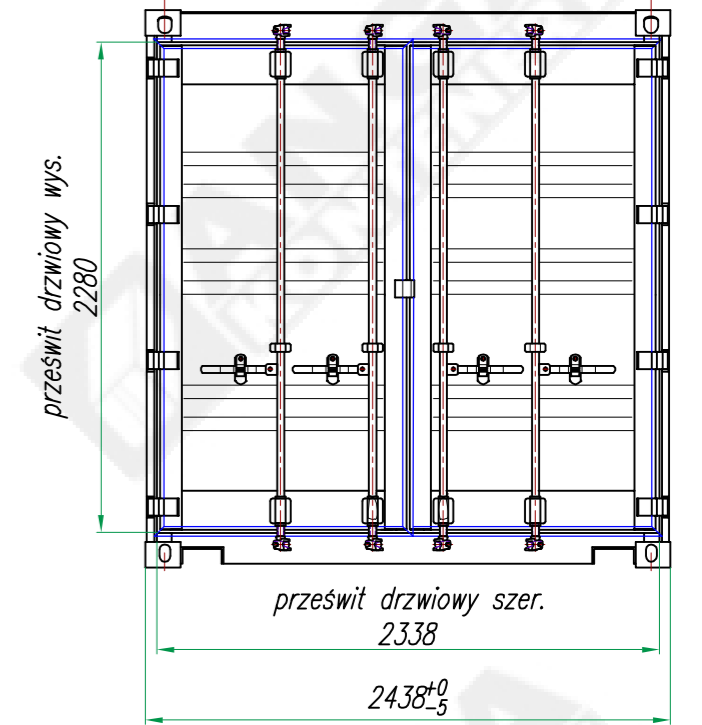
Widok B
