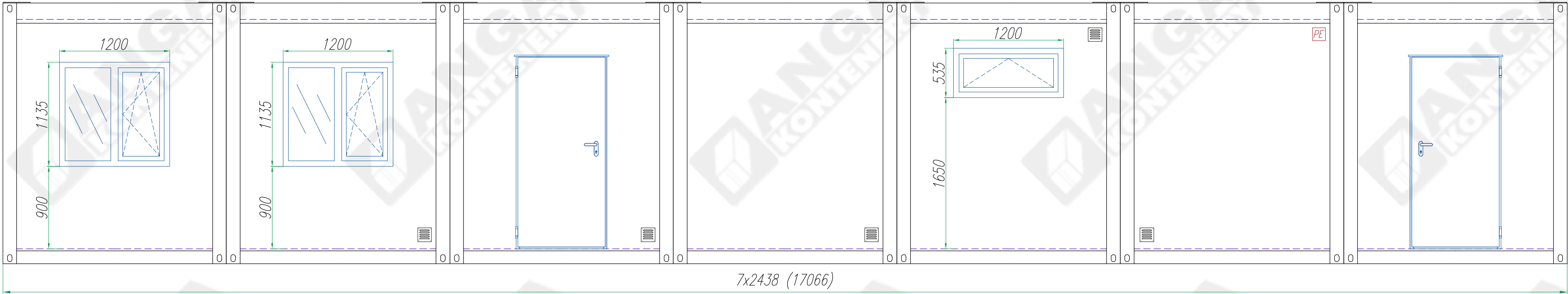
Widok B
