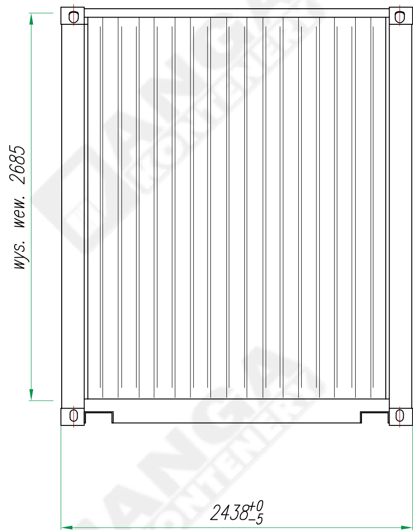
Widok C
