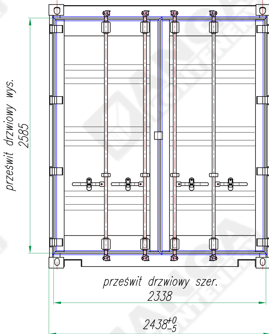
Widok B
