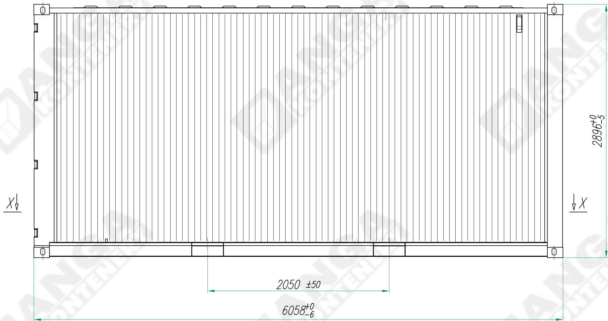
Widok A
